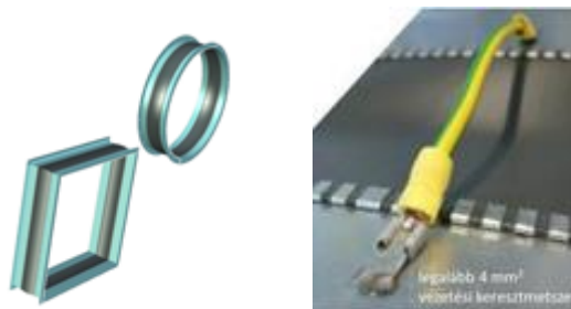
F-1. ábra: légszűrőbe építendő hőtágulási kompenzátorok; potenciálkiegyenlítés
